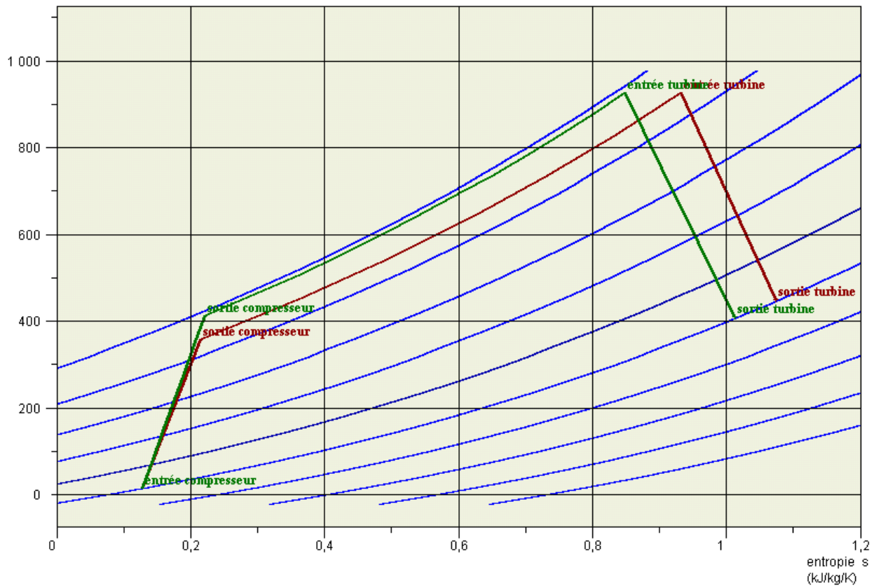
diagramme entropique (T,s) : air
